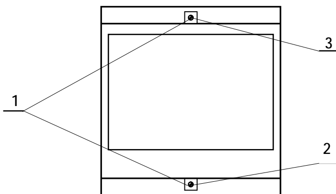
Рисунок 2 – Общий вид ИП в корпусе с габаритными размерами 60×85×75 мм
