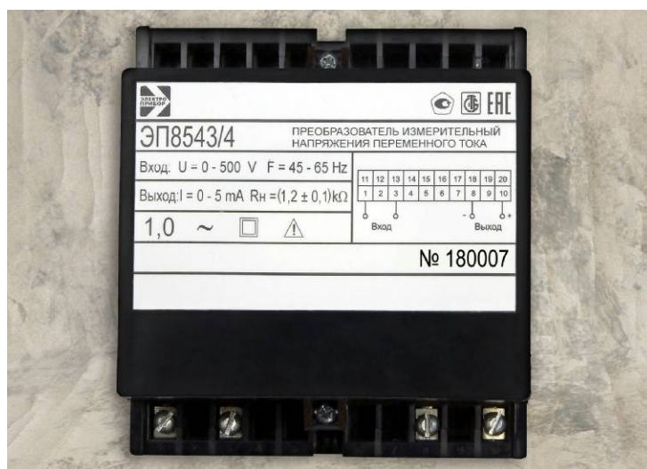
Рисунок 1 – Общий вид ИП в корпусе с габаритными размерами 110×120×70 мм (при креплении на винты) или 110×120×81 мм (при креплении на DIN – рейку)
