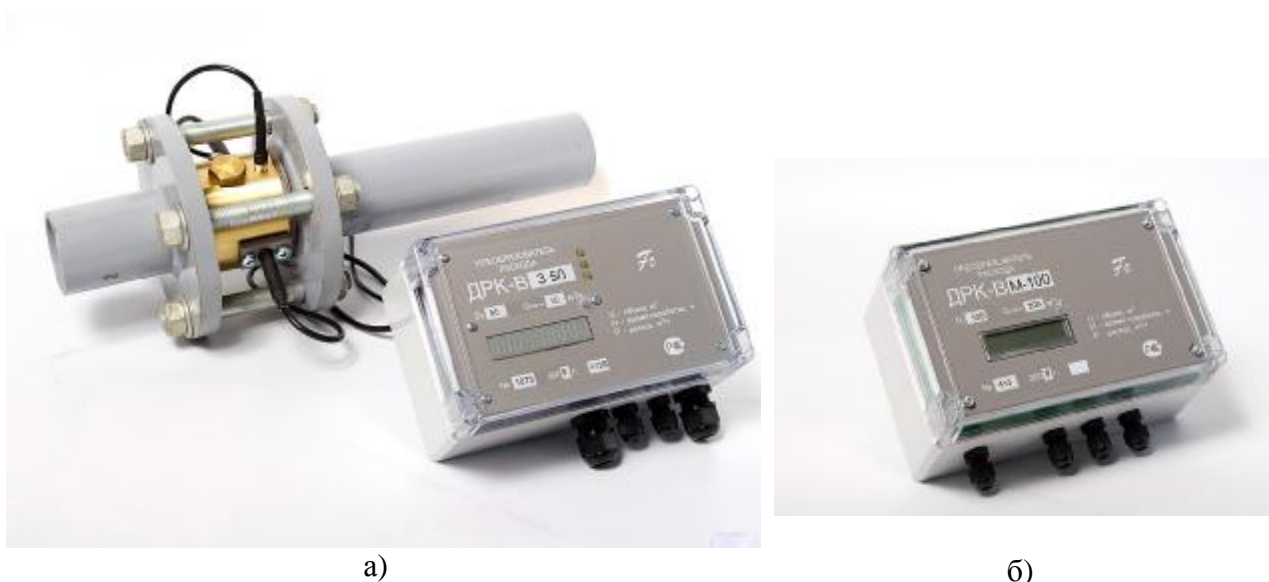
Рисунок 1 - Внешний вид расходомера жидкости корреляционного вихревого ДРК-В: а) модификация ДРК-В3, б) электронный преобразователь модификации ДРК-ВМ
