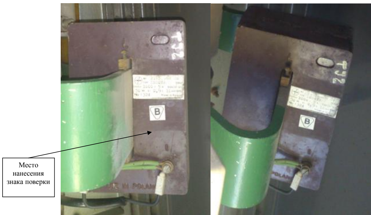
Рисунок 1 - Фотография внешнего вида трансформаторов ISZOTA
