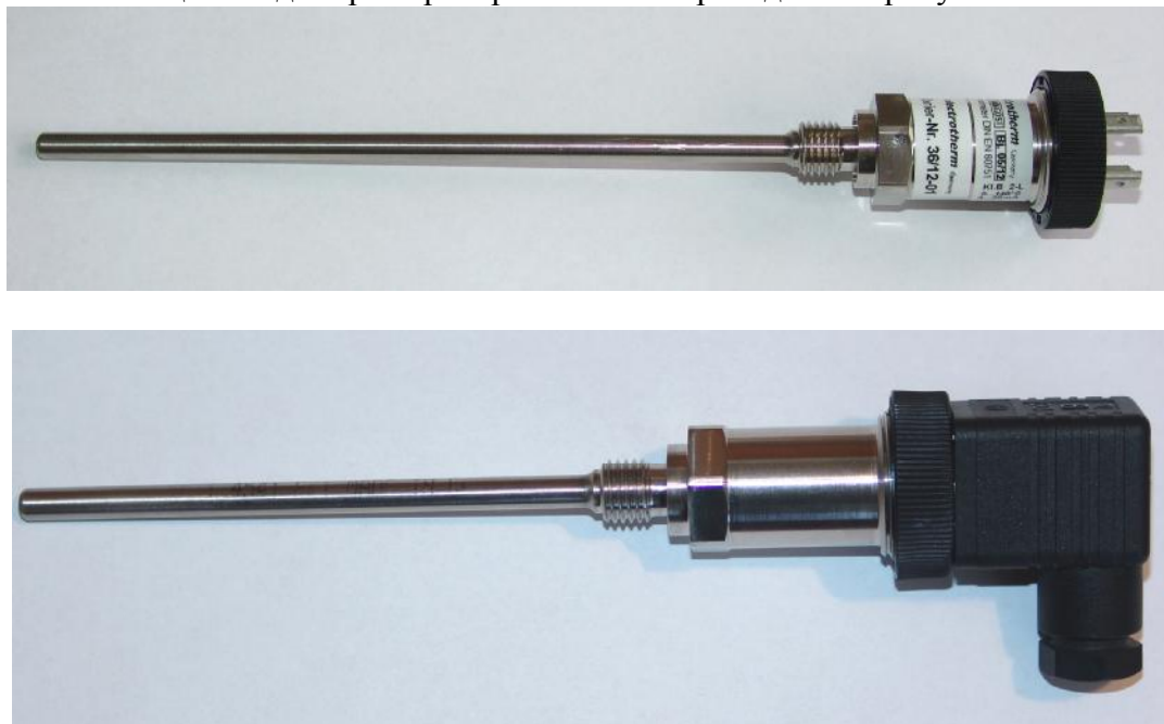
Рис. 1. Термопреобразователи сопротивления с унифицированным выходным сигналом 406GOST.
