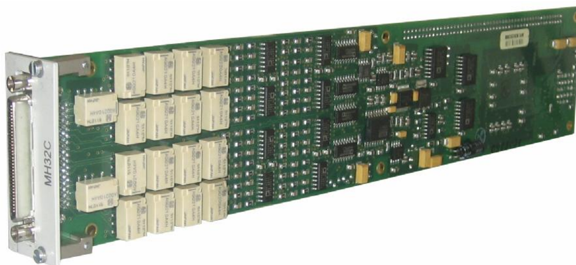
Рисунок 5 – Внешний вид измерителя MH32C ФТКС.468266.019
