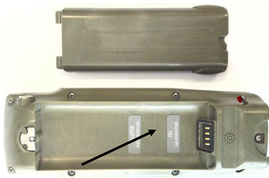
Рисунок 2 – Место нанесения знака об утверждении типа
