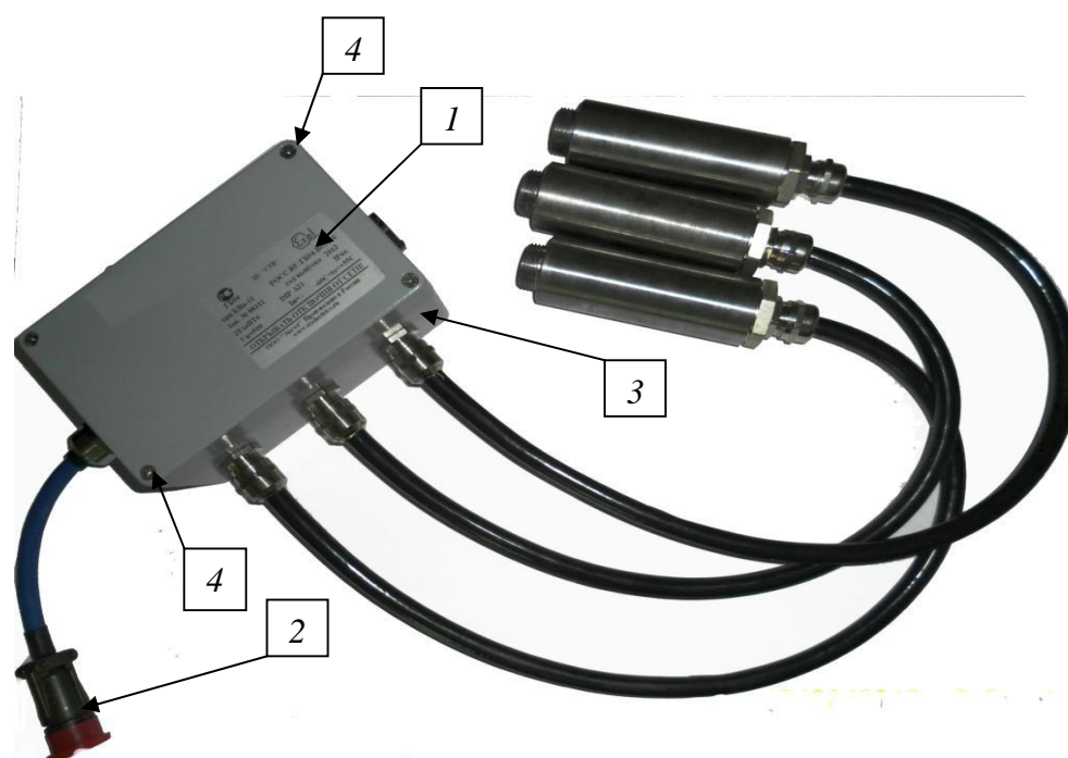
Рис. 2. Внешний вид регистратора РГГ-2.
