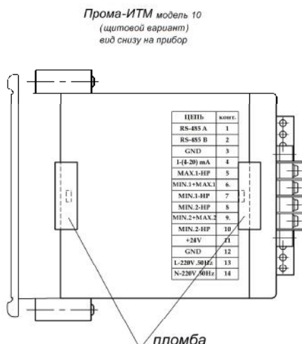
Рис.1. Схема пломбировки измерителя ПРОМА-ИТМ
