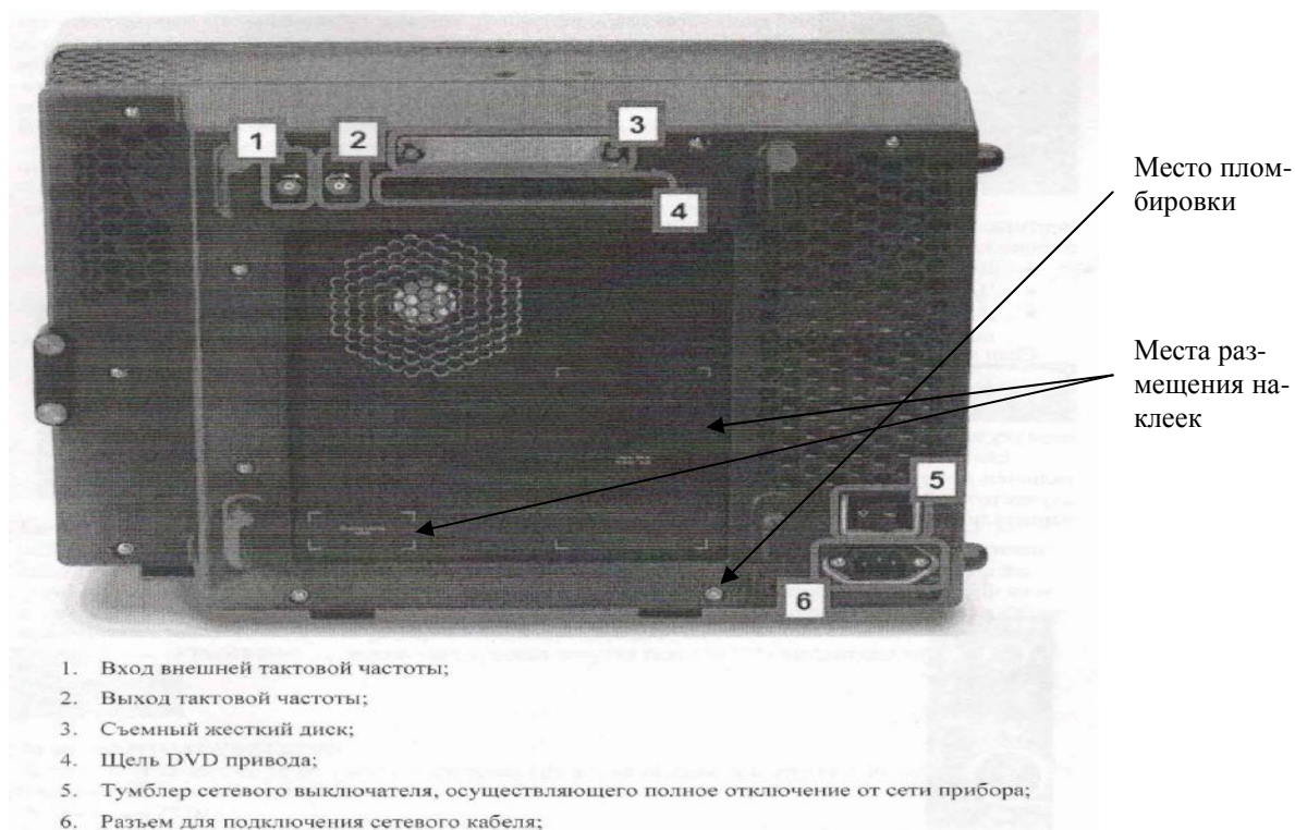
Рисунок 3 - Схемы для размещения наклеек и пломбировки от несанкционированного доступа
