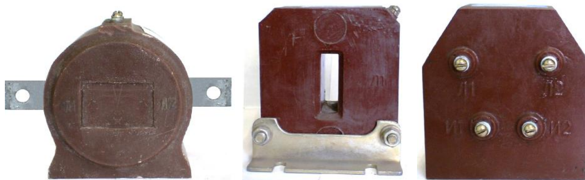
Рисунок 1 – Фотография общего вида трансформаторов тока ТКС-0,66, ТШС-0,66, ТРС-0,66
