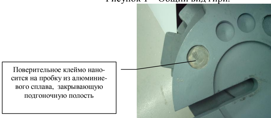
Рисунок 2 – Схема пломбирования от несанкционированного доступа и обозначение мест для нанесения клейма.
