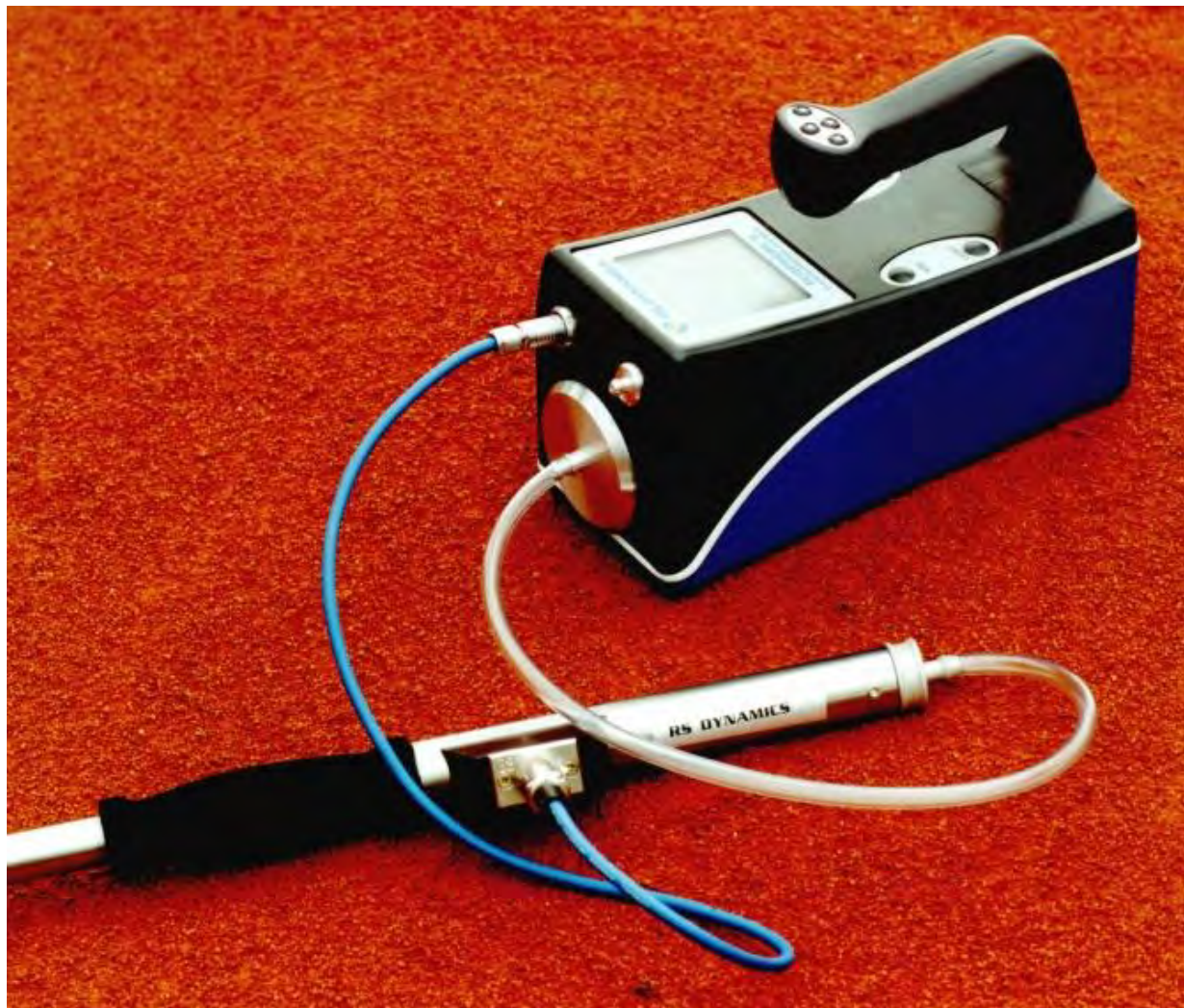
Рис. 1 Общий вид газоанализатора ESCOProbe 5
