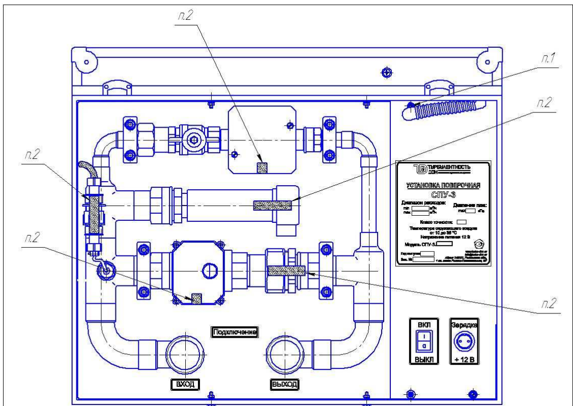
Рисунок 3 - Схема пломбирования установок
