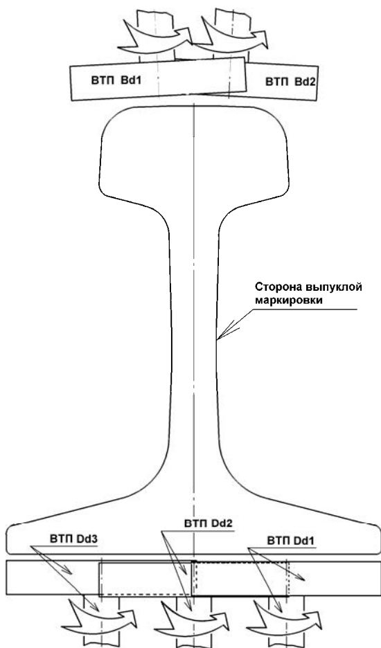
Рисунок 2 – Динамические ВТП
