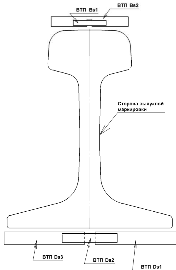
Рисунок 3 – Статические ВТП
