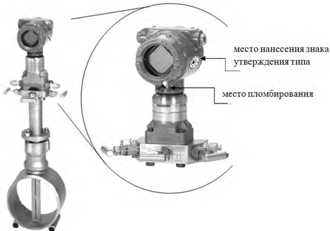
Фото общего вида расходомеров 3051SFA
