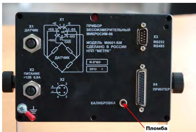
Рисунок 4 - Схема пломбировки весов монорельсовых M8700
