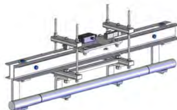
Рисунок 2 – Вид модификации М8700-2
