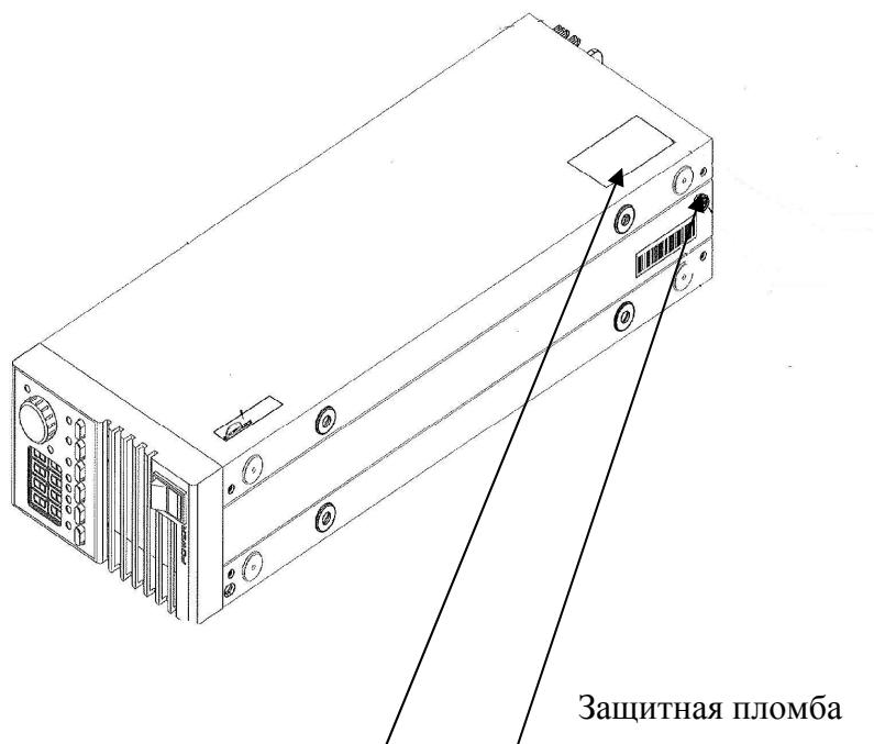
Рисунок 2 – Схема пломбирования
