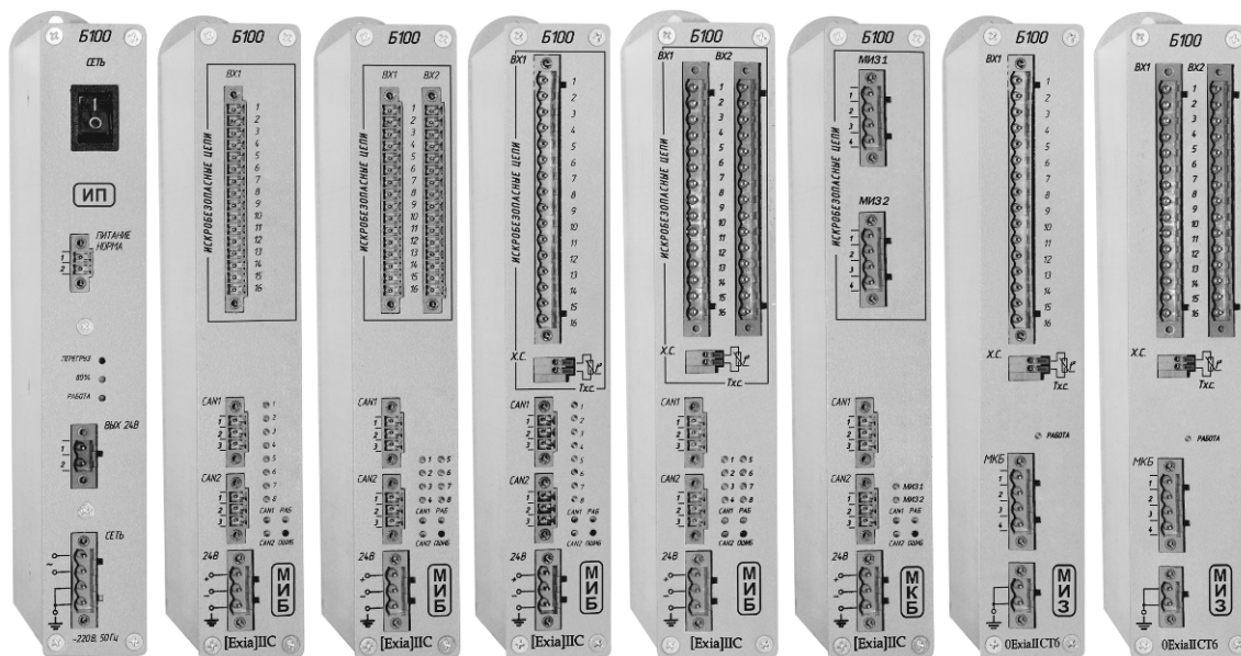
Рисунок 1 — Общий вид контроллера БАЗИС-100
