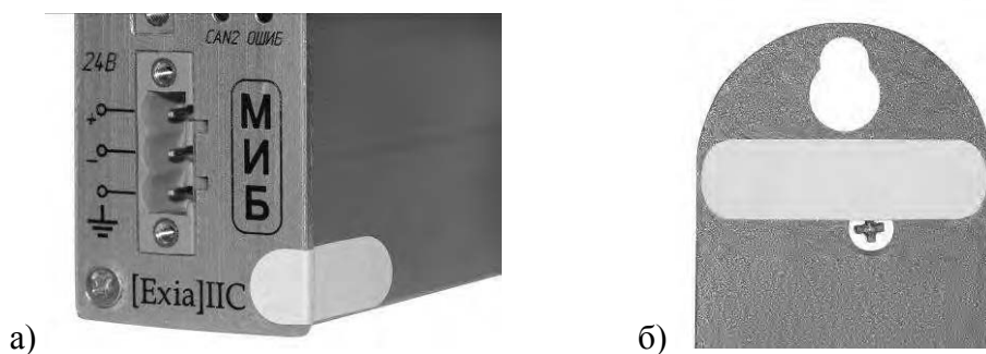
Рисунок 2 — Пломбирование измерительных модулей контроллера БАЗИС-100: а) пломбирование передней панели; б) пломбирование задней панели
