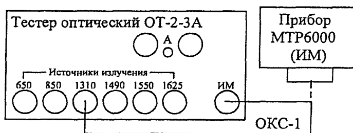
ИМ - измеритель мощности, ОКС-1 – кабель оптический соединительный Рисунок 11
