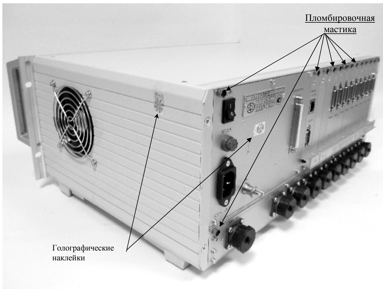
Рисунок 2. Схема пломбировки от несанкционированного доступа, обозначения мест для нанесения оттисков клейм и нанесения наклеек
