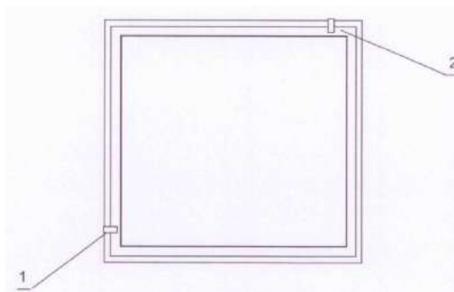
Рисунок 2 - Схема пломбировки от несанкционированного доступа и указание мест размещения клейм-наклеек ОТК и знака поверки средств измерений для модификаций ЦП8507/1, ЦП8507/2, ЦП8507/7, ЦП8507/8 (1 - клеймо-наклейка ОТК, 2 - клеймо-наклейка знака поверки средств измерений)
