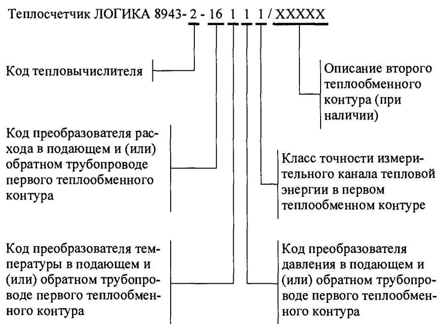
Рисунок 2.1 – Структура обозначения теплосчетчиков
