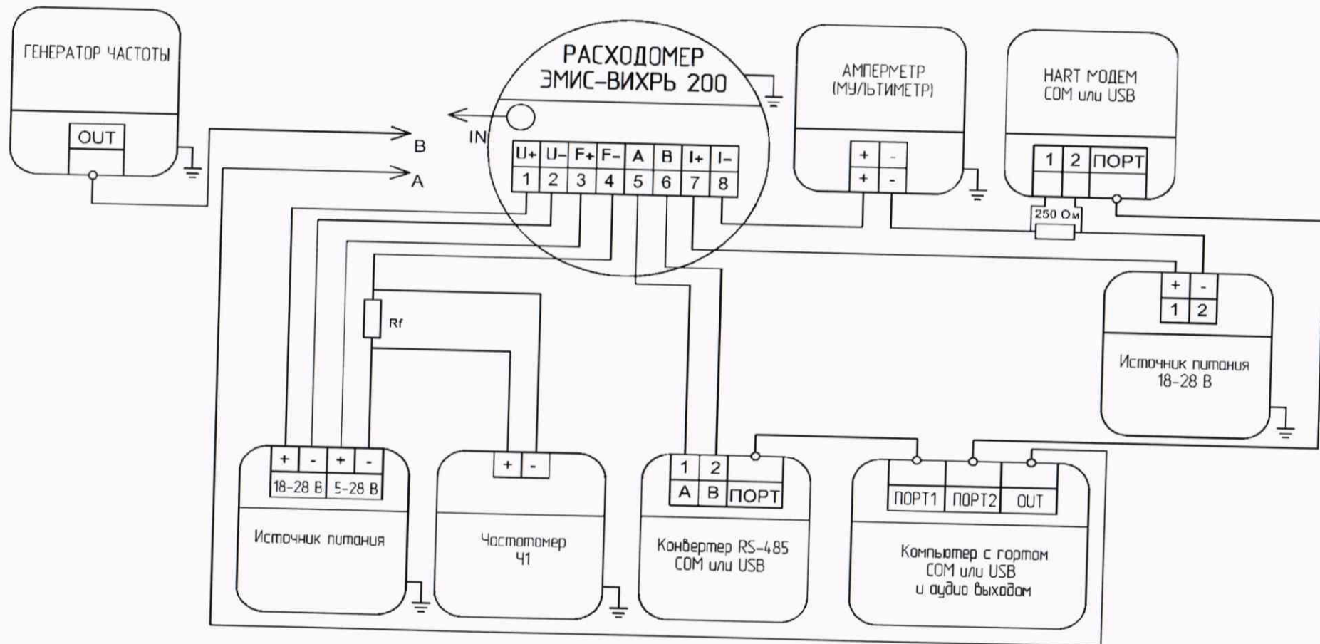
Рисунок А.1 – Схема подключения расходомеров при определении метрологических характеристик имитационным способом
