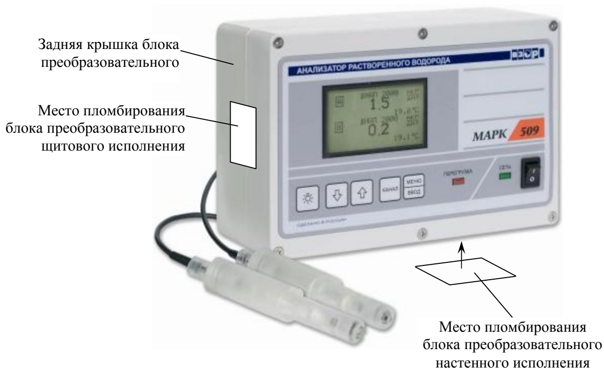
Рисунок – Анализатор растворенного водорода МАРК-509
