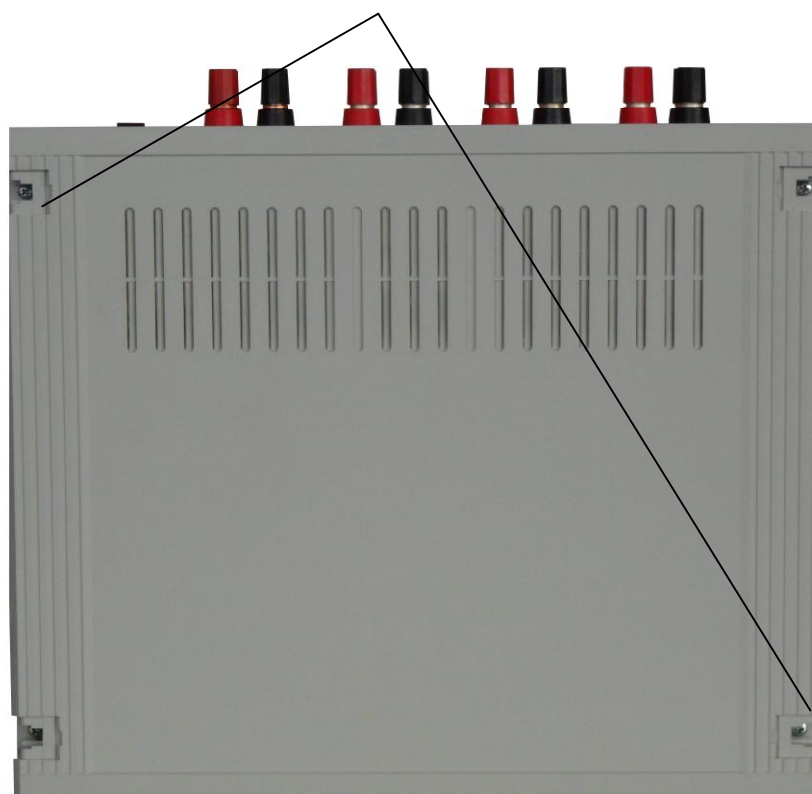
Рисунок 2 - Места нанесения поверительного клейма
