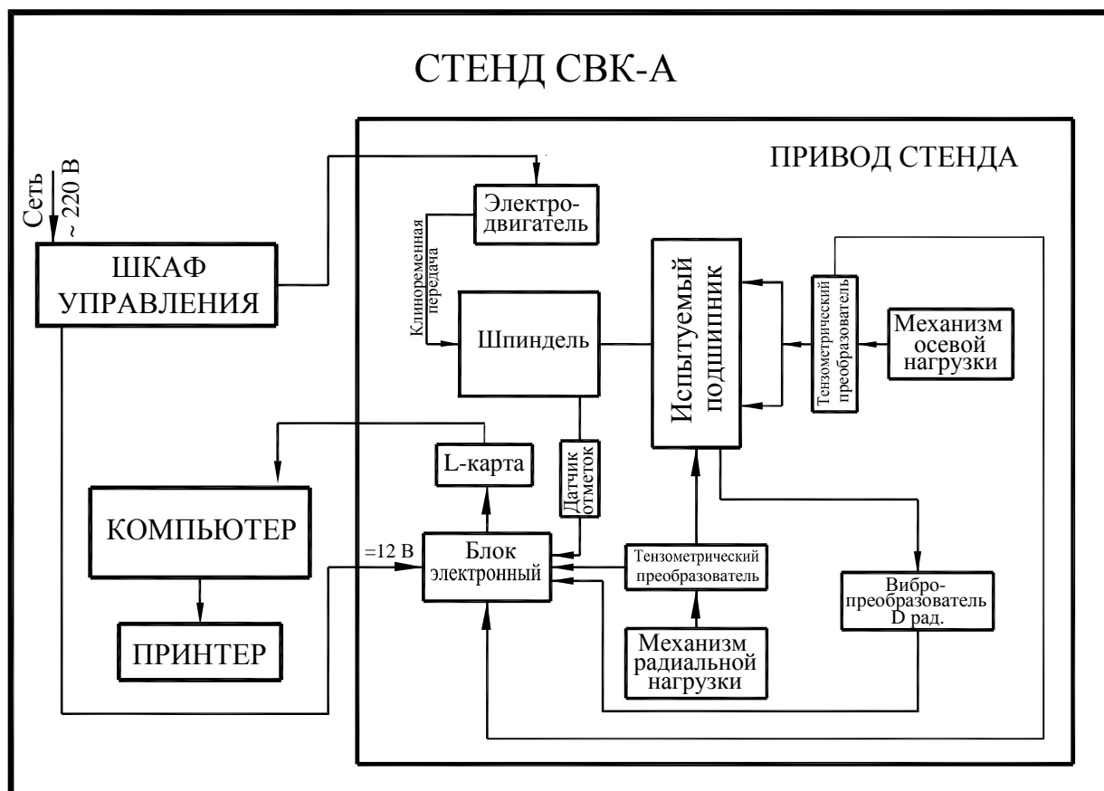
Рисунок 2 – Структура стенда вибрационного контроля подшипников СВК-А
