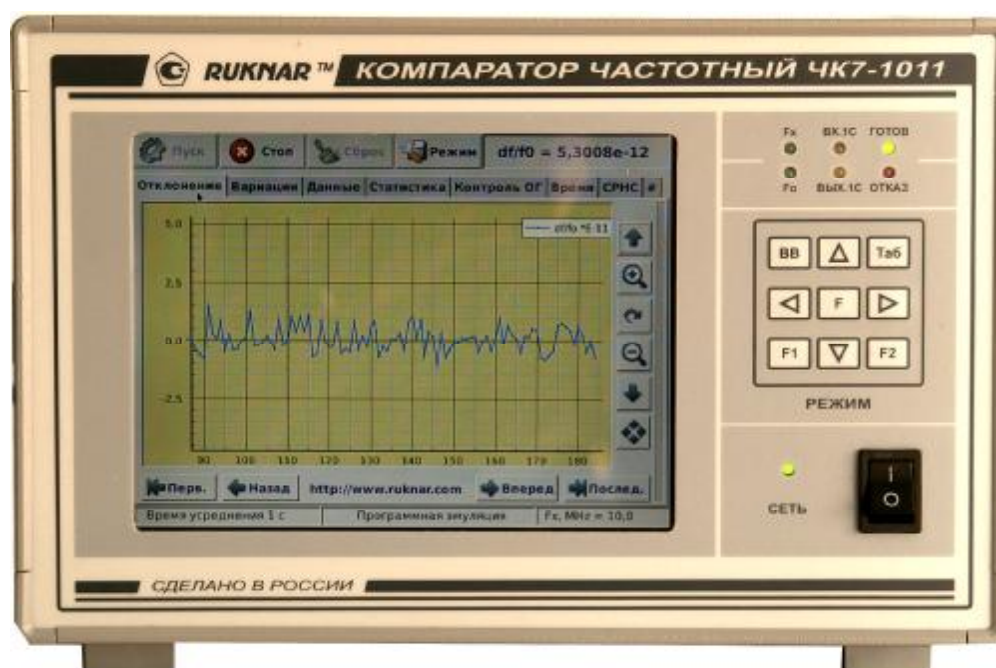
Рисунок 1 – Общий вид компараторов.
