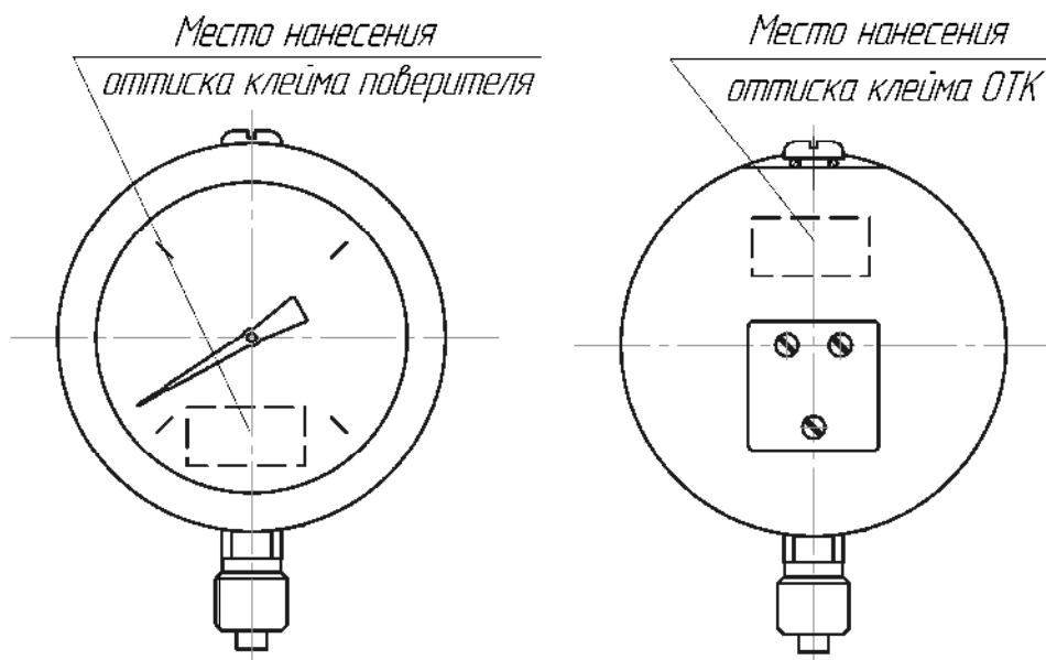
Рисунок 2 - Схема обозначения мест для нанесения оттисков клейм
