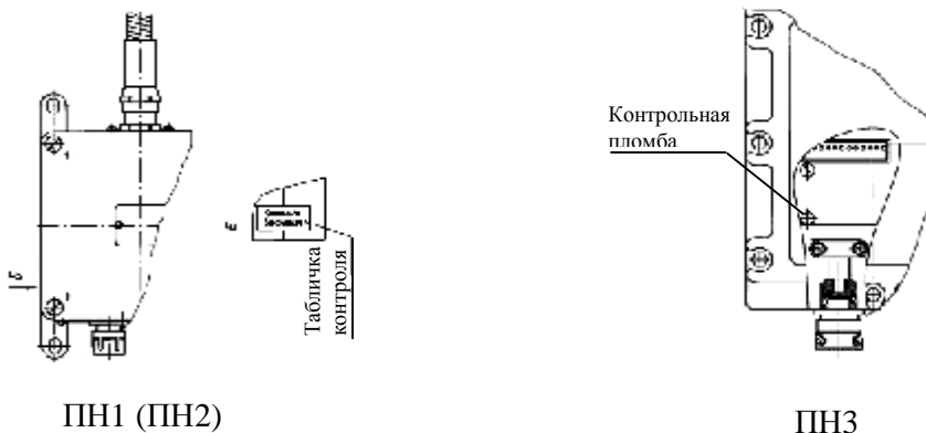
Схема пломбировки от несанкционированного доступа
