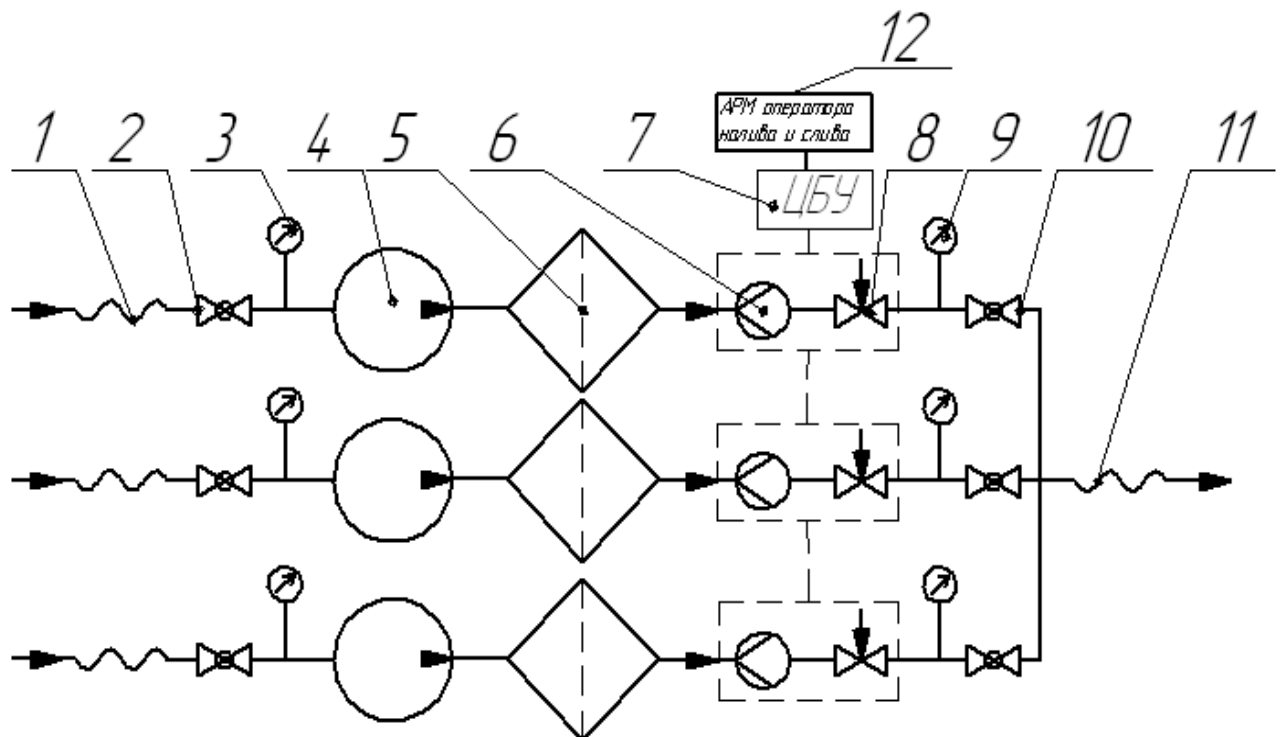
1, 11-компенсатор трубопроводов; 2, 10-кран шаровой; 3- мановакуумметры; 4-насос; 5- фильтр жидкости; 6-счетчик; 7-вторичный прибор; 6-клапан управляемый; 9-манометр, 12- АРМ оператора налива и слива.
