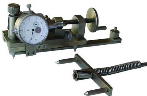
Рисунок 1 – Общий вид измерителя
