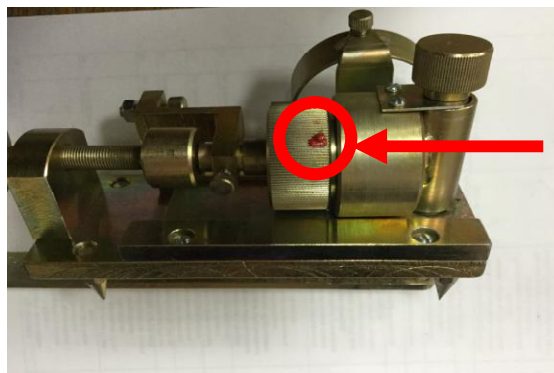
Рисунок 2 – Место пломбировки от несанкционированного доступа
