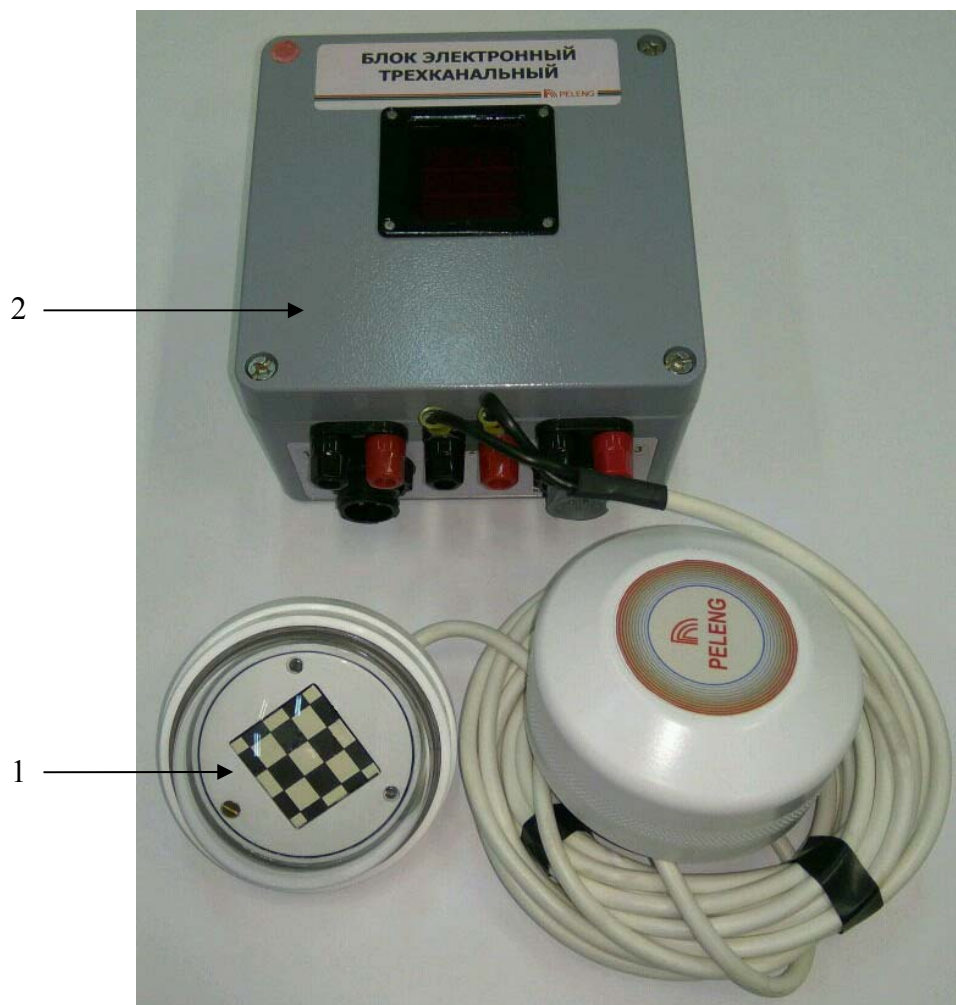
Рисунок 1 - Общий вид пиранометров «Пеленг СФ-06» 1 - головка пиранометра, 2 - блок электронный трехканальный
