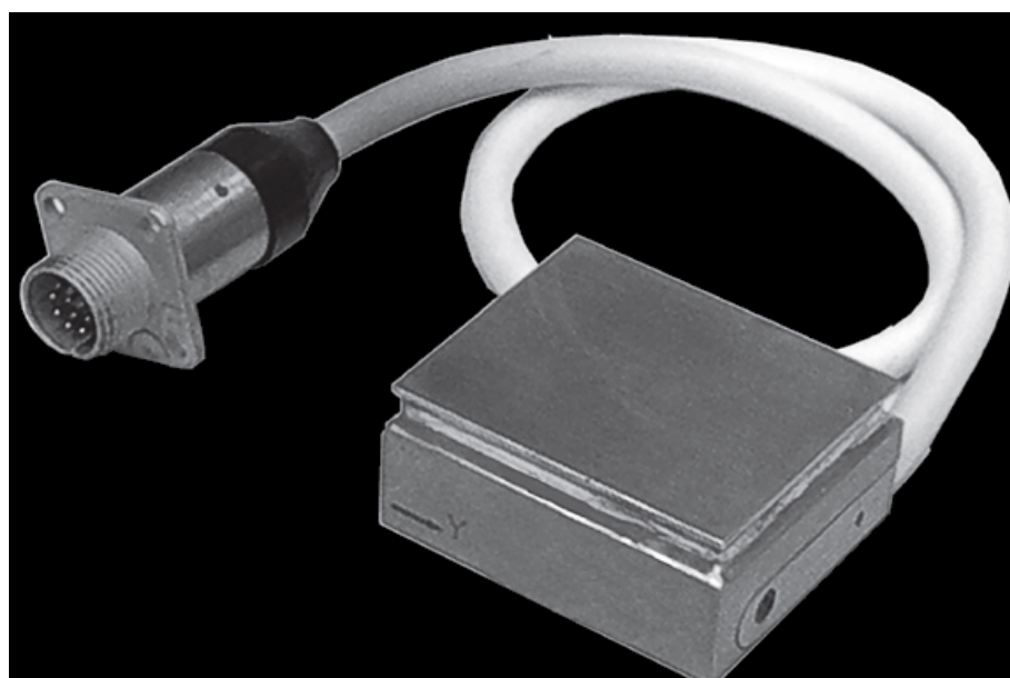
Рисунок 1 – Общий вид акселерометра
