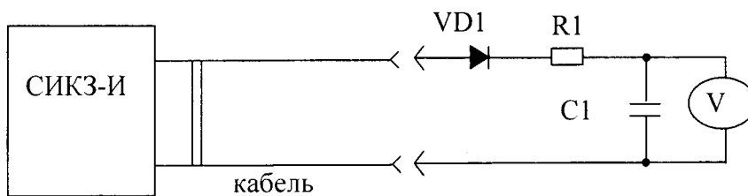
Рисунок А.2 – Схема измерения выходного напряжения сигнализаторов СИКЗ-И (всех исполнений) СИКЗ-Е, СИКЗ-Р-И(II) (в случае, если переключки установлены для работы с клапаном импульсного напряжения питания)
