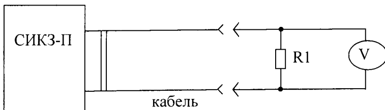
Рисунок А.3 – Схема измерения выходного напряжения сигнализаторов СИКЗ-П (всех исполнений), СИКЗ-Р-И(II) (в случае, если переключки установлены для работы с клапаном постоянного напряжения питания)
