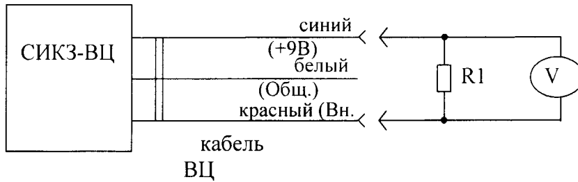
Рисунок А.1 – Схема измерения выходного напряжения сигнализаторов СИКЗ-ВЦ (всех исполнений)
