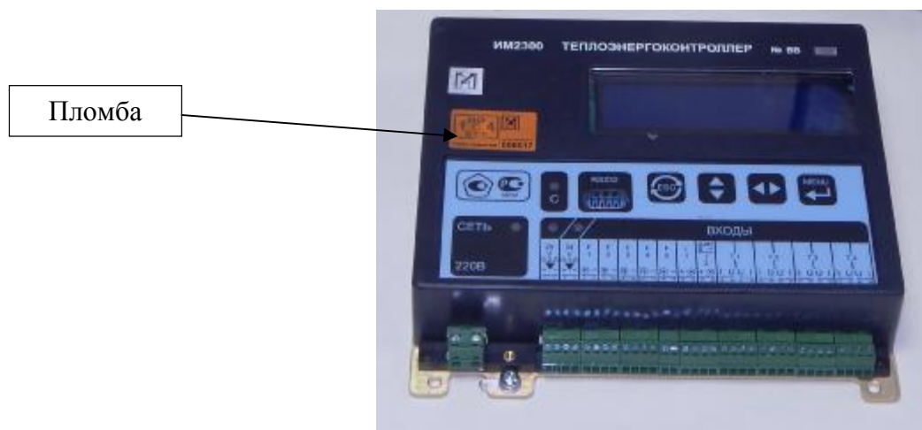
Рисунок 2 - Схема пломбировки теплосчетчиков ИМ2300Т
