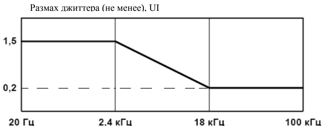
Рисунок 2 - Максимально допустимый размах джиттера входного сигнала тестера
