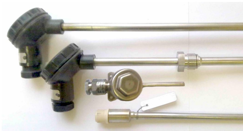
Рисунок 1 - Общий вид термопреобразователей сопротивления ТСП-01
