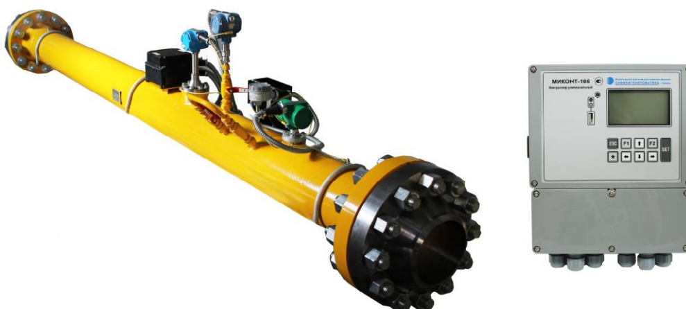
Рисунок 4 - Счетчик газа вихревой ИК-СВГ.МЗ-200
