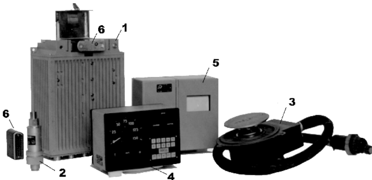
Рисунок 1 – Общий вид КПД-3В
