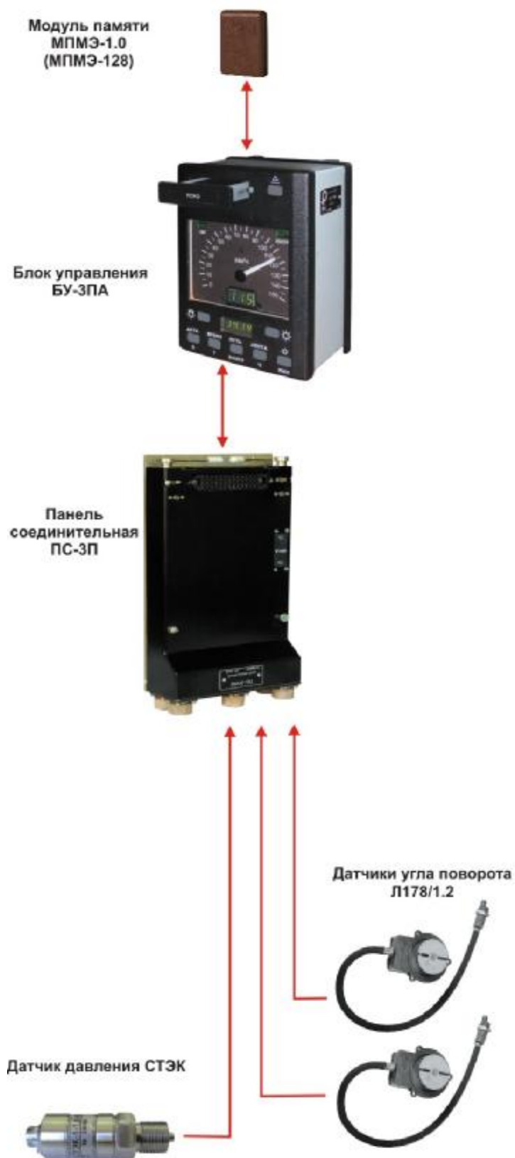
Рисунок 3 – Общий вид КПД-3ПА
