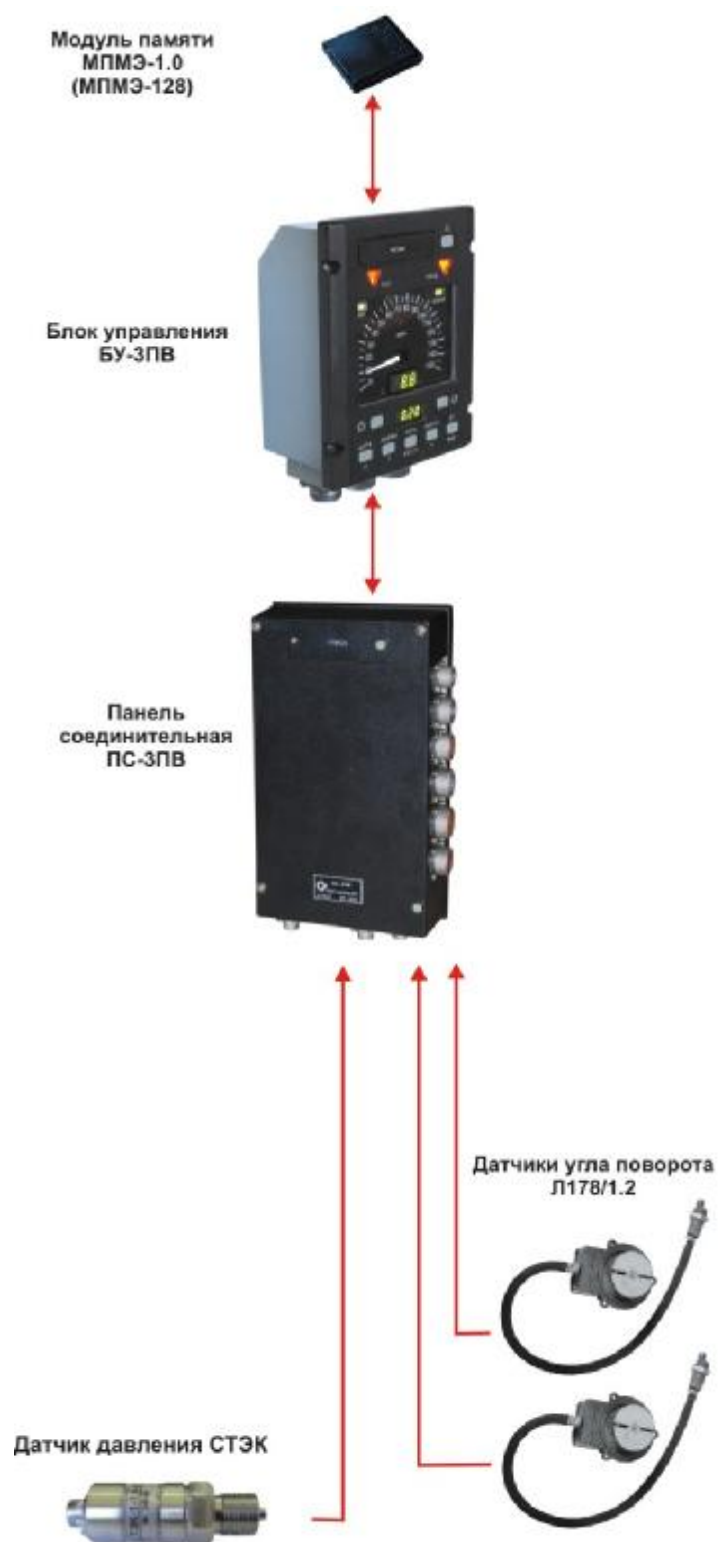
Рисунок 4 – Общий вид КПД-ЗПВ
