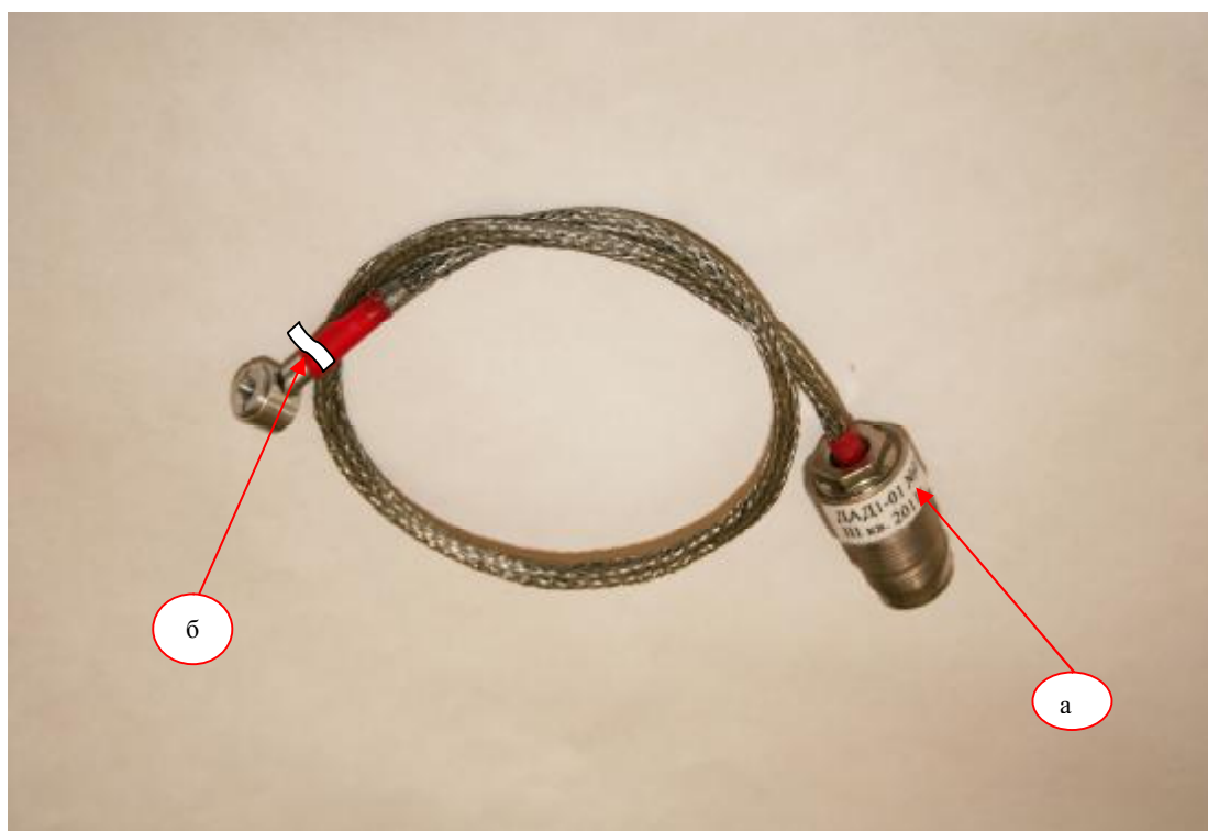
Рисунок 4 – Место нанесения наклейки (а) и пломбировки (б) детектора ДАД1-01
